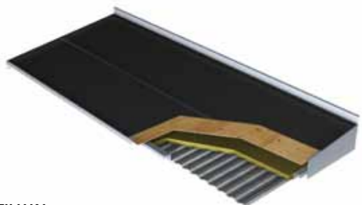
C. TILLVAL Stomme av varmförzinkad stål, isolerad med invändig takplåt av trapetskorrugerad aluzinkplåt och utvändig plyfa samt duk/papp.
