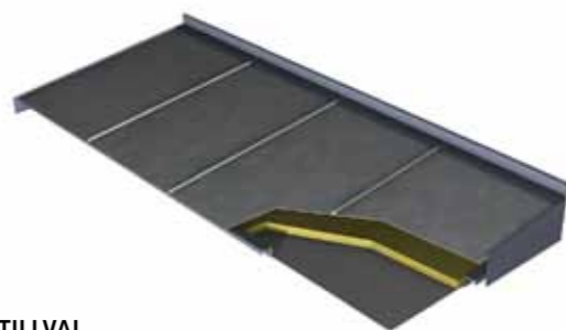
B. TILLVAL Integrerad takram av aluminium. Taktäckning med ThermiSol isolerelement – skivans utsida är svart, insidan är vit.
