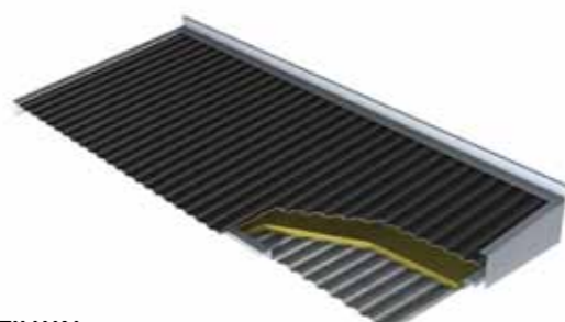
D. TILLVAL Stomme av varmförzinkad stål, isolerad och med in- och utvändig takplåt av trapetskorrugerad aluzinkplåt.
